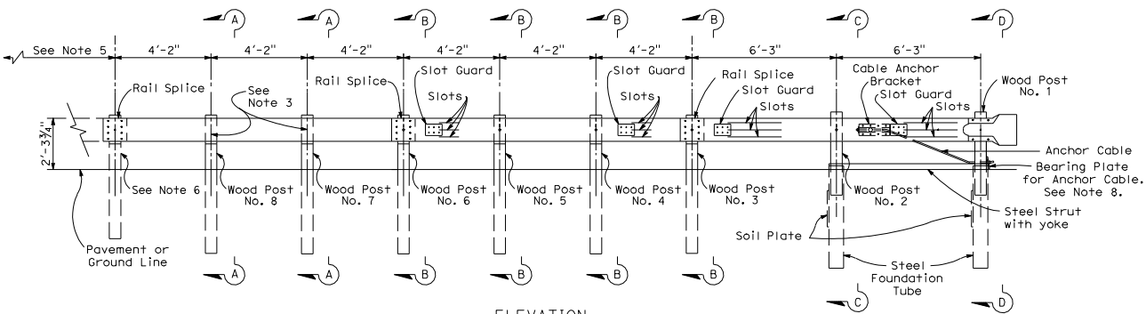
ELEVATION
